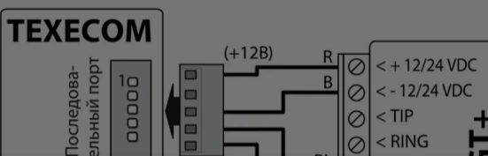
Схема подключения охранной панели TEXECOM
